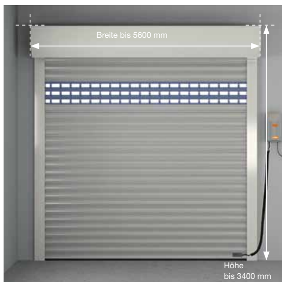
Rolltor ROLENTO: Die maximale Breite ist abhängig von der Torhöhe. Ihr Fachbetrieb zeigt Ihnen die Möglichkeiten.
