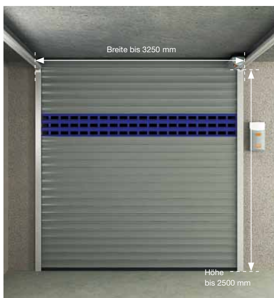
Deckenlauftor GECCO von ROMA ist bestens geeignet für Einzelgaragen mit begrenzten Einbauverhältnissen.
