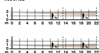
Empfindlicher Bereich des Infrarotsensors - SEITENANSICHT
