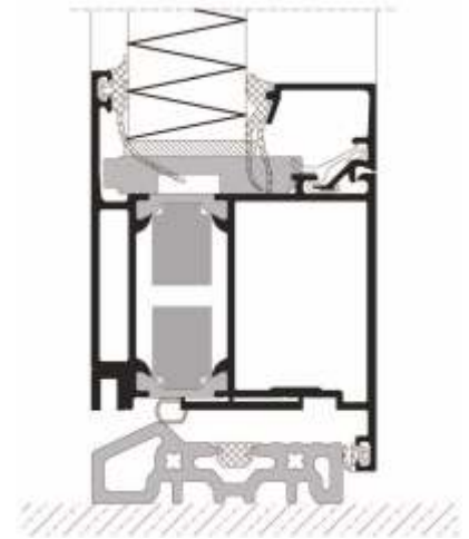
Standard-ECO-Konstruktion als 106mm hoher Fußpunkt mit umlaufendem Flügel (in der Höhe nicht einstellbar)
