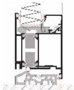
günstige ECO-Konstruktion als 106mm hoher Fußpunkt mit umlaufenden Flügel (nicht einstellbar)
